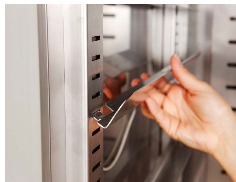
Crémaillère inox 74 positions
