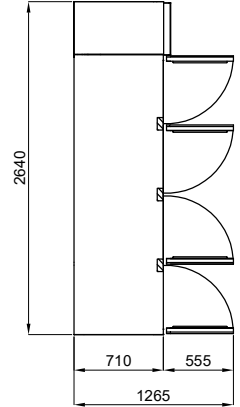
PART. INGOMBRO PORTE SCALA 1 : 60
