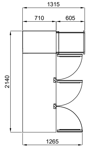
PART. INGOMBRO PORTE SCALA 1 : 50
