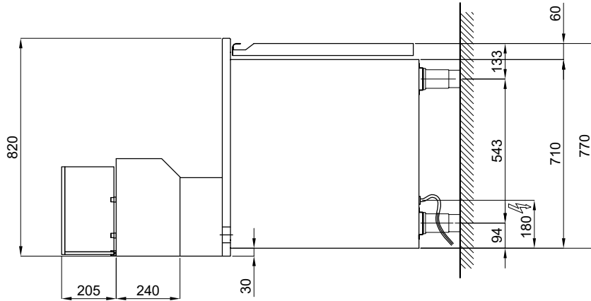
PART. INGOMBRO PORTE SCALA 1 : 50
