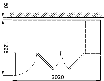
PART. INGOMBRO PORTE SCALA 1 : 50
